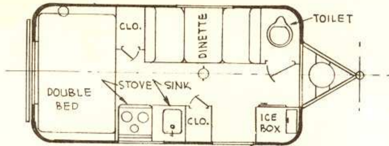
17' CHICO
